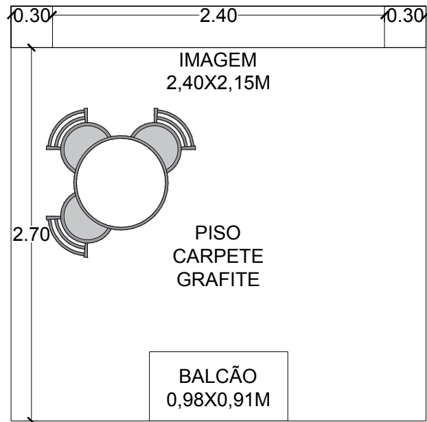
PLANTA BAIXA
